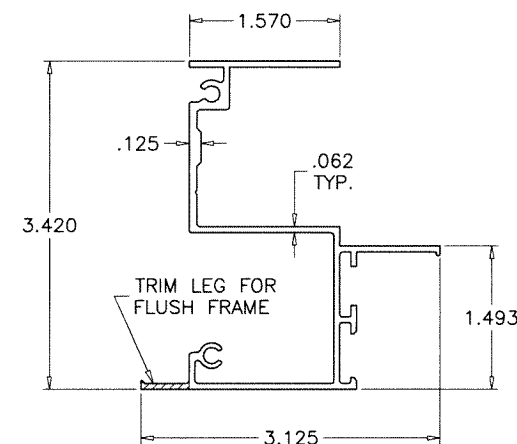
3 FRAME JAMB
